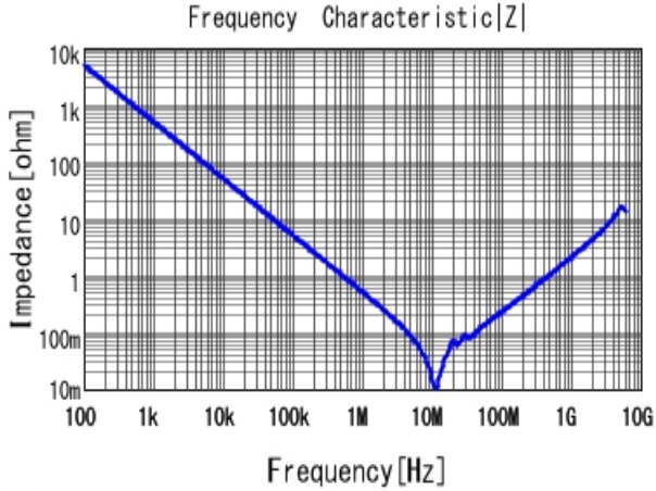
■ GRM21BR71E334KA01 |Z| DCOV, 25degC
