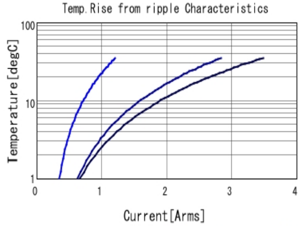
GRM21BR71E334KA01 Temp. rise ■ 100kHz ■ 500kHz ■ 1MHz
