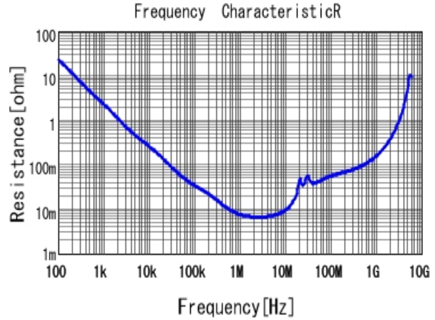
■ GRM21BR71E334KA01 R DCOV, 25degC
