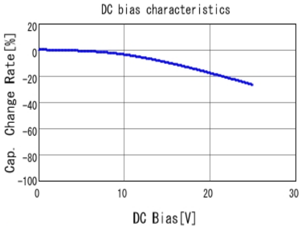
■ GRM21BR71E334KA01 C-DC bias capchange, 25.0degC, AC1.
