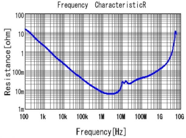
■ GRM21BR71E225KE11 R DCOV, 25degC
