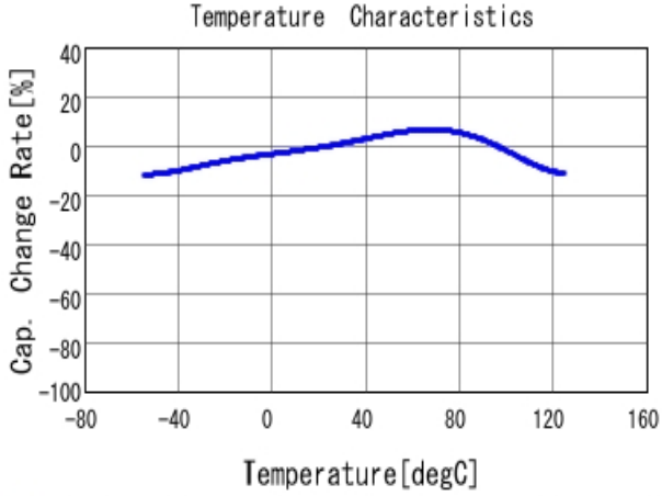
■ GRM21BR71E225KE11 C-Temp. capchange, DCO. 0V, ACO. 8Vrm
