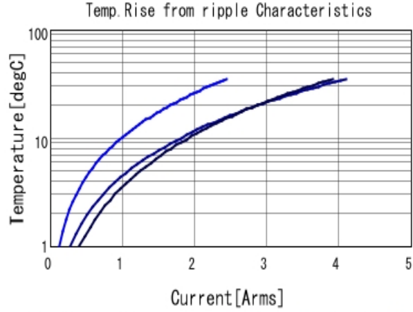
GRM21BR71E225KE11 Temp. rise ■ 100kHz ■ 500kHz ■ 1MHz
