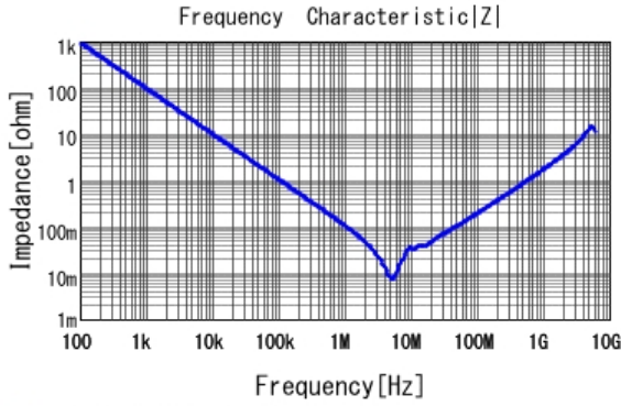
■ GRM21BR71E225KA73 |Z| DCOV, 25degC
