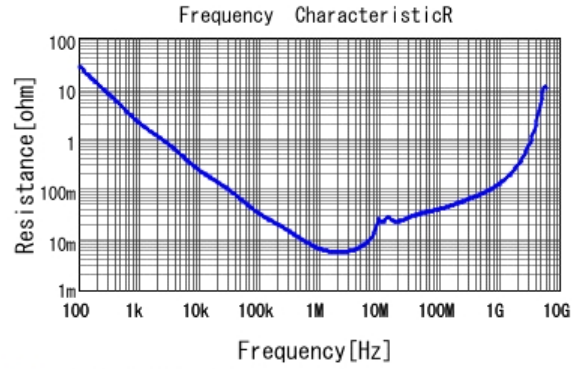
■ GRM21BR71E225KA73 R DCOV, 25degC
