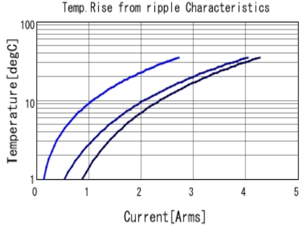
GRM21BR71A475KA73 Temp. rise ■ 100kHz ■ 500kHz ■ 1MHz
