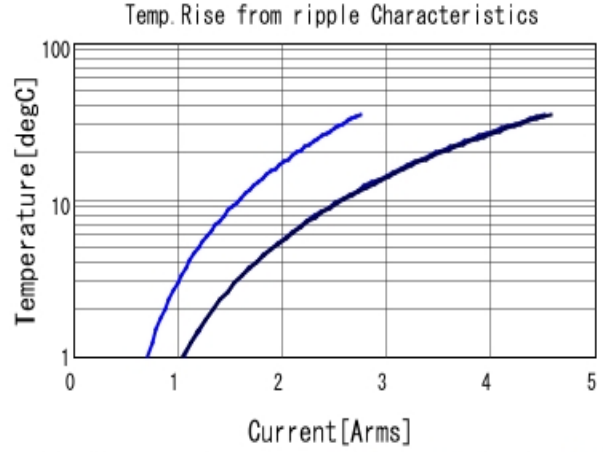
GRM21BR71A225MA01 Temp. rise ■ 100kHz ■ 500kHz ■ 1MHz
