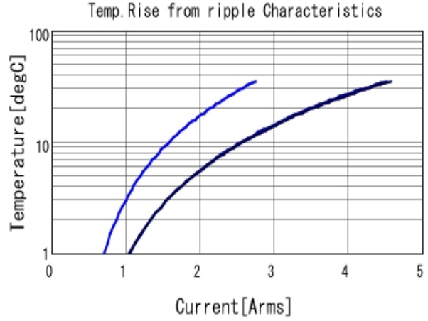
GRM21BR71A225KA01 Temp. rise ■ 100kHz ■ 500kHz ■ 1MHz
