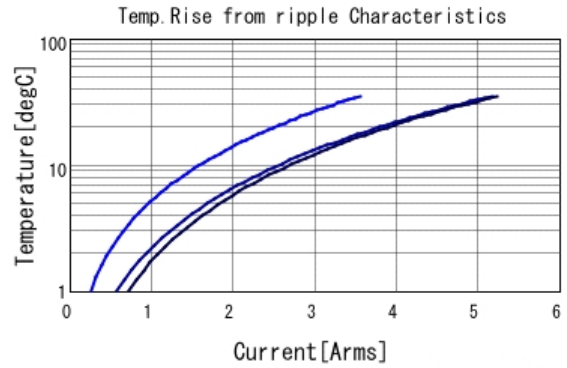
GRM21BR71A106MA73 Temp. rise ■ 80kHz ■ 400kHz ■ 800kHz
