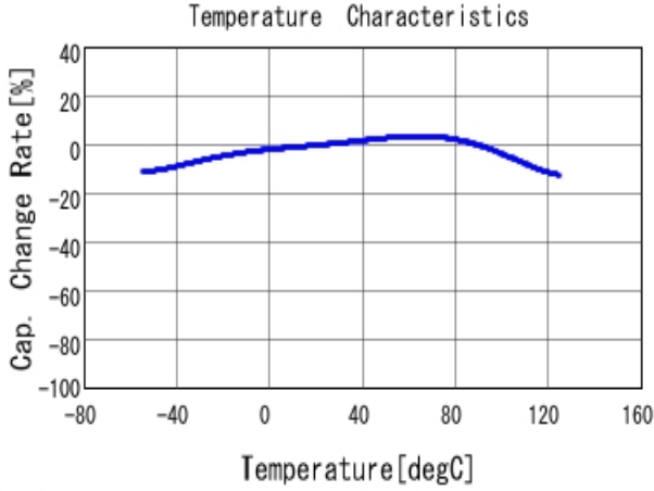
■ GRM21BR71A106KA73 C-Temp. capchange, DCO. 0V, ACO. 35Vr
