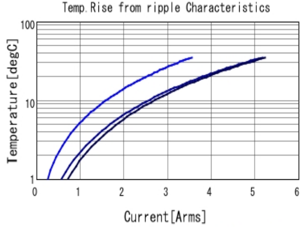
GRM21BR71A106KA73 Temp. rise ■ 80kHz ■ 400kHz ■ 800kHz
