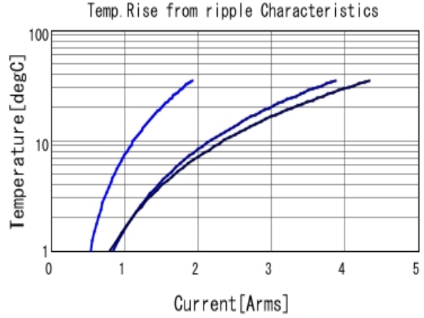
GRM21BR71A105KA01 Temp. rise ■ 100kHz ■ 500kHz ■ 1MHz
