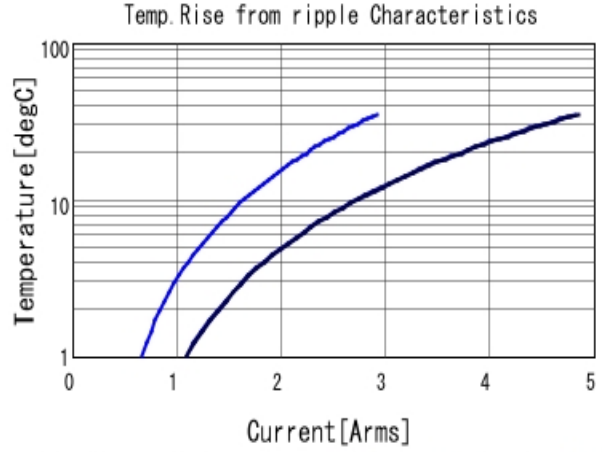
GRM21BR70J225KA01 Temp. rise ■ 100kHz ■ 500kHz ■ 1MHz
