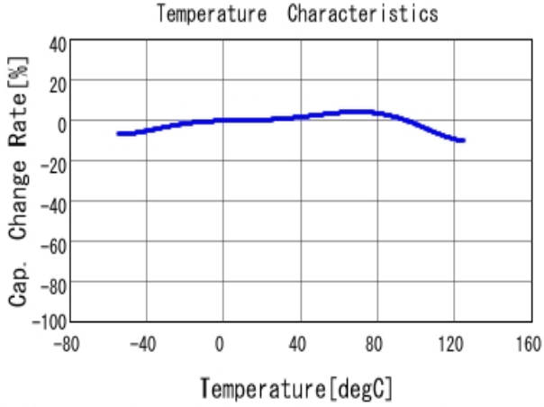
■ GRM21BR70J106KE76 C-Temp. capchange, DCO. 0V, ACO. 5Vrm
