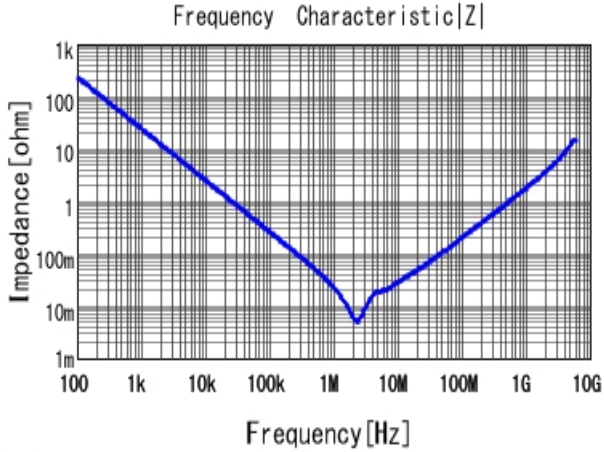
■ GRM21BR70J106KE76 |Z| DCOV, 25degC
