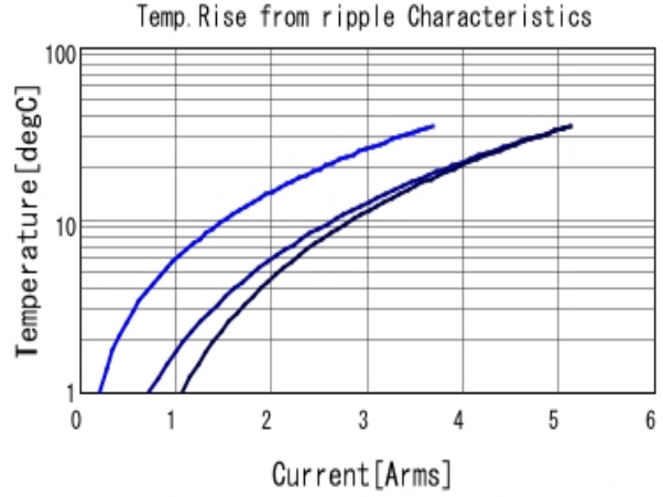
GRM21BR70J106KE76 Temp. rise ■ 80kHz ■ 400kHz ■ 800kHz
