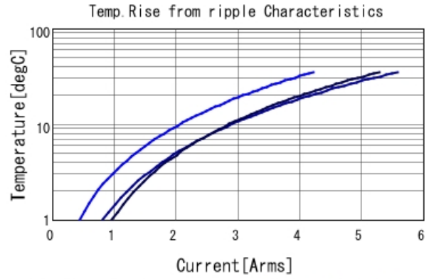
GRM21BR6YA106ME43 Temp. rise ■ 80kHz ■ 400kHz ■ 800kHz
