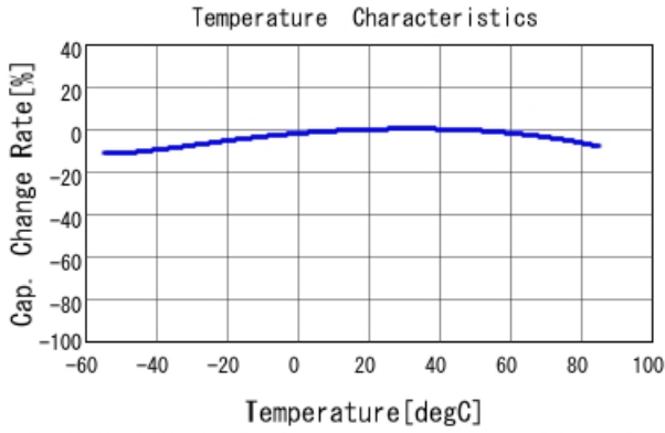
■ GRM21BR6YA106ME43 C-Temp. capchange, DCO. 0V, ACO. 5Vrm
