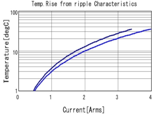
GRM21BR61H225KA73 Temp. rise ■ 500kHz ■ 1MHz
