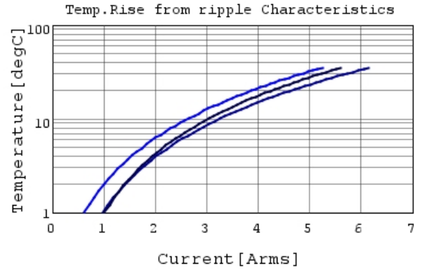
GRM21BR61E226ME44 Temp.rise — 80kHz —
