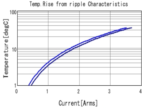
GRM21BR61E225KA12 Temp. rise ■ 500kHz ■ 1MHz
