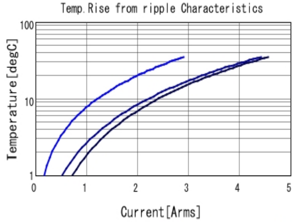
GRM21BR61C475KA88 Temp. rise ■ 100kHz ■ 500kHz ■ 1MHz
