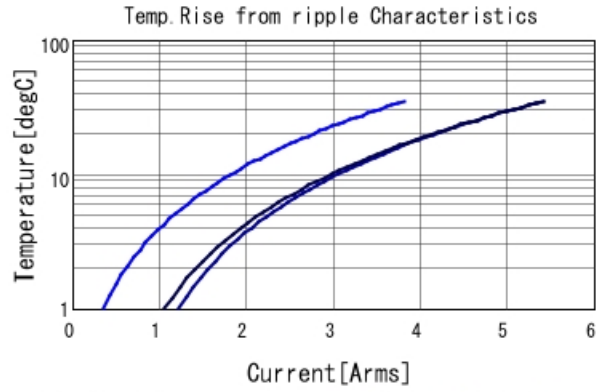
GRM21BR61C106ME15 Temp. rise ■ 80kHz ■ 400kHz ■ 800kHz
