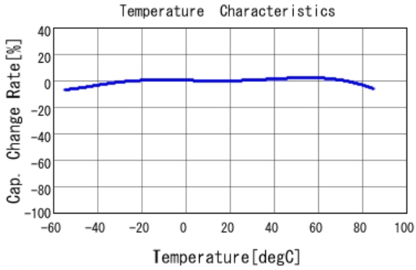
■ GRM21BR61C106ME15 C-Temp. capchange, DCO. 0V, ACO. 5Vrm
