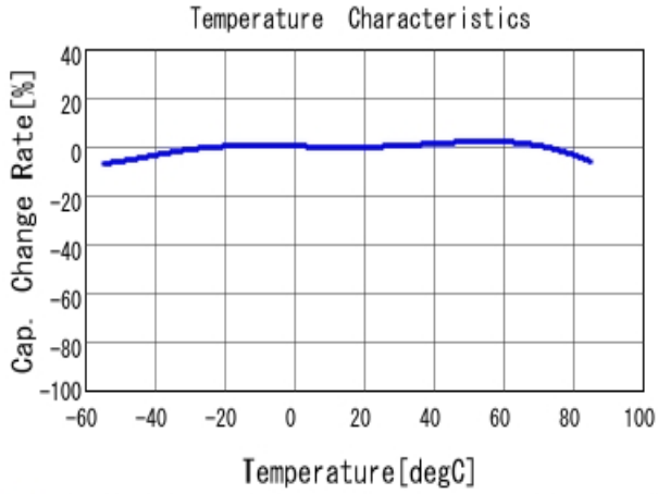
■ GRM21BR61C106KE15 C-Temp. capchange, DCO. 0V, ACO. 5V rm
