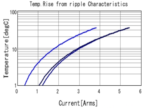
GRM21BR61C106KE15 Temp. rise ■ 80kHz ■ 400kHz ■ 800kHz
