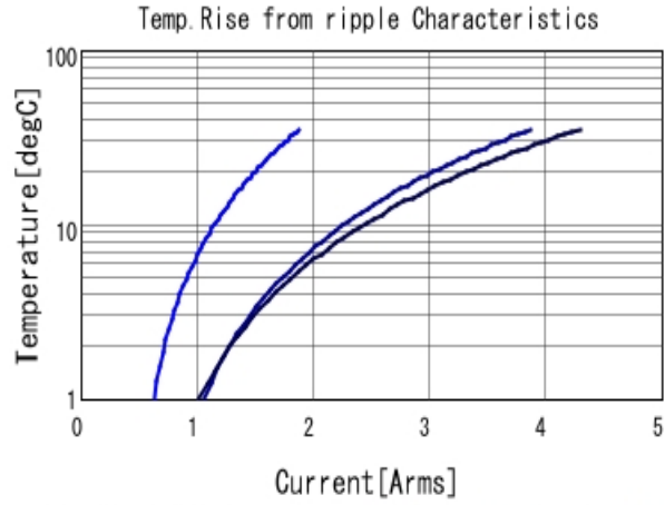
GRM21BR61C105KA01 Temp. rise ■ 100kHz ■ 500kHz ■ 1MHz
