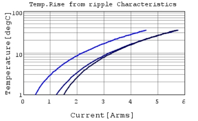
GRM21BR60J226ME39 Temp.rise — 80kHz —
