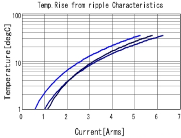
GRM21BD71A226ME44 Temp. rise ■ 80kHz ■ 400kHz ■ 800kHz
