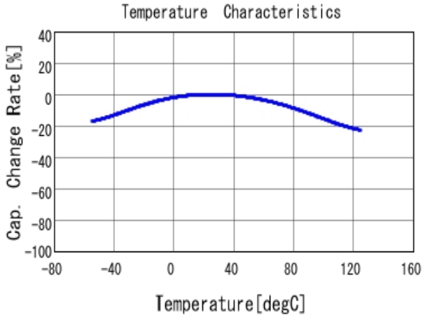
■ GRM21BD71A226ME44 C-Temp. capchange, DCO. 0V, ACO. 1Vrm
