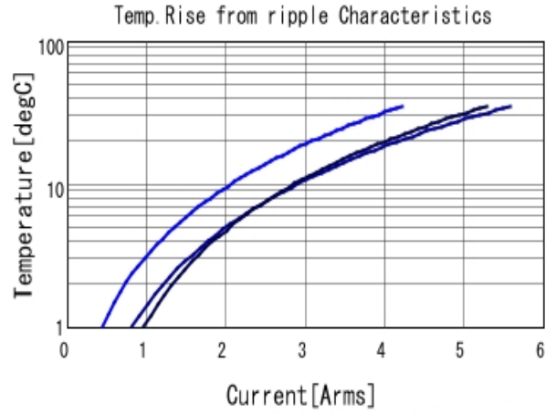
GRM21BC8YA106KE11 Temp. rise ■ 80kHz ■ 400kHz ■ 800kHz
