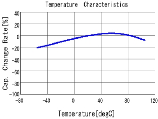
■ GRM21BC8YA106KE11 C-Temp. capchange, DCO. 0V, ACO. 2V rm
