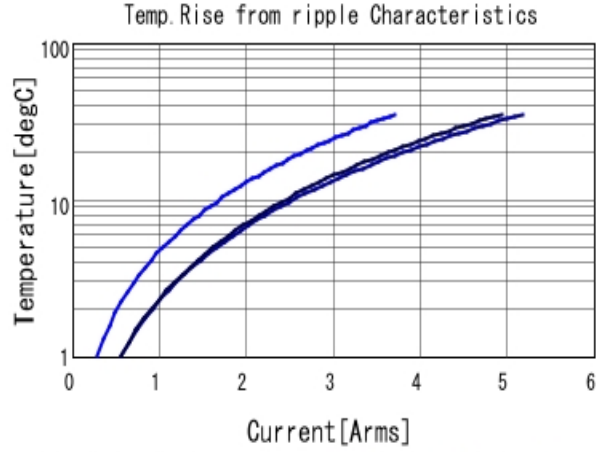
GRM21BC81E106KE51 Temp. rise ■ 80kHz ■ 400kHz ■ 800kHz
