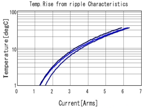
GRM21BC80G476ME15 Temp. rise ■ 60kHz ■ 300kHz ■ 600kHz
