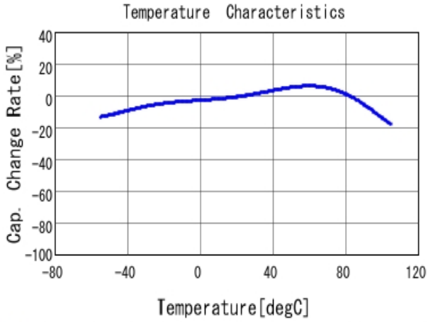
■ GRM21BC80G476ME15 C-Temp. capchange, DCO. 0V, ACO. 1Vrm
