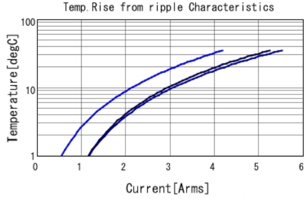
GRM21BC71E106ME11 Temp. rise ■ 80kHz ■ 400kHz ■ 800kHz
