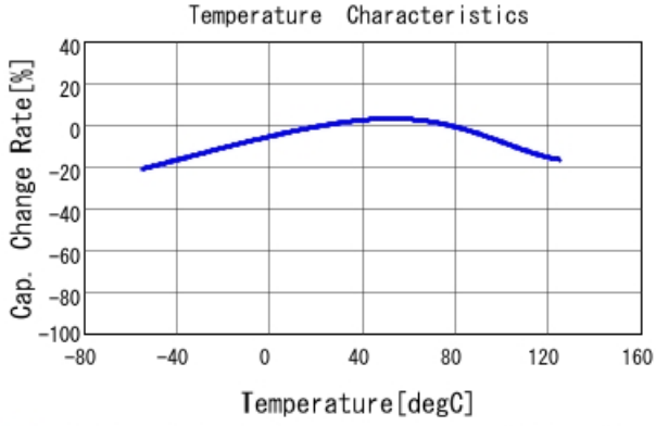
■ GRM21BC71E106ME11 C-Temp. capchange, DCO. 0V, ACO. 2Vrm
