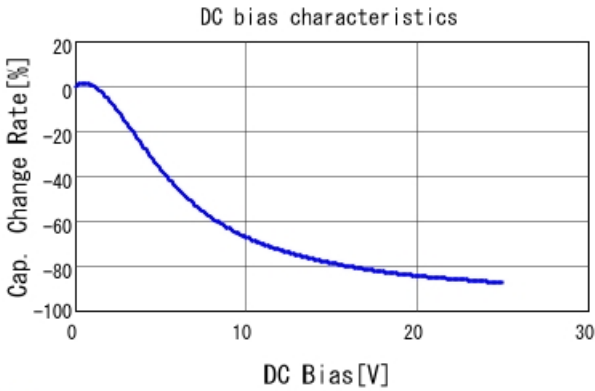
■ GRM21BC71E106ME11 C-DC bias capchange, 25.0degC, AC1V
