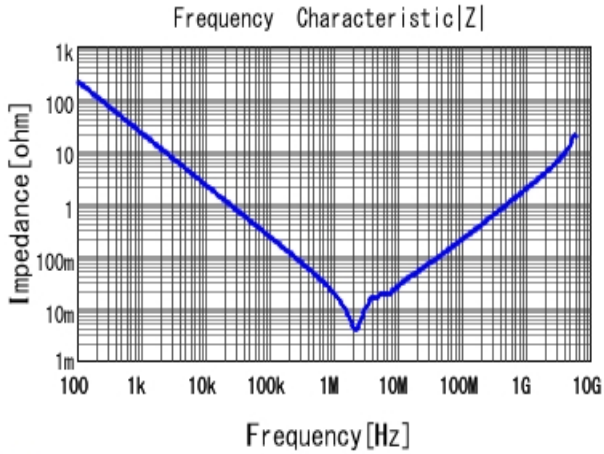
■ GRM21BC71E106KE11 |Z| DCOV, 25degC
