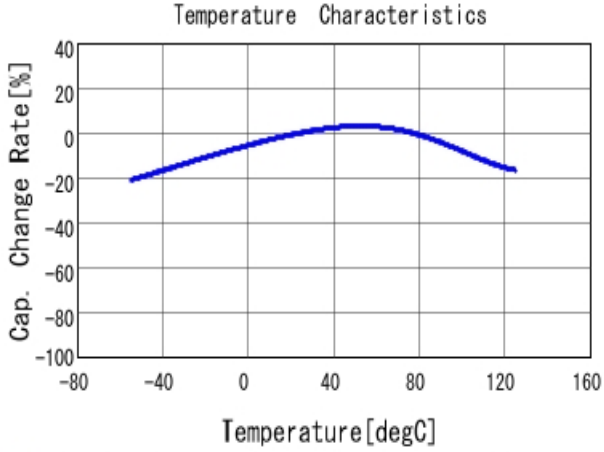
■ GRM21BC71E106KE11 C-Temp. capchange, DCO. 0V, ACO. 2V rm
