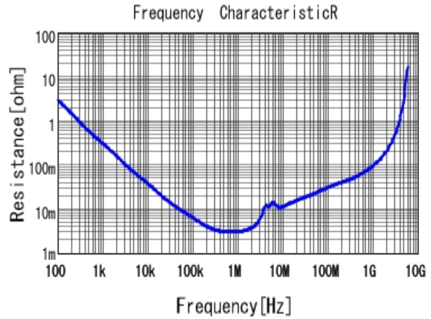
■ GRM21BC71E106KE11 R DCOV, 25degC
