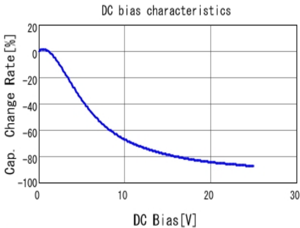
■ GRM21BC71E106KE11 C-DC bias capchange, 25.0degC, AC1V
