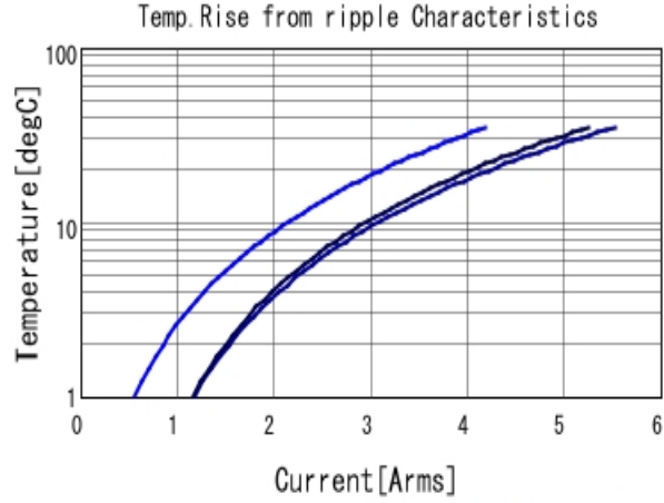
GRM21BC71E106KE11 Temp. rise ■ 80kHz ■ 400kHz ■ 800kHz
