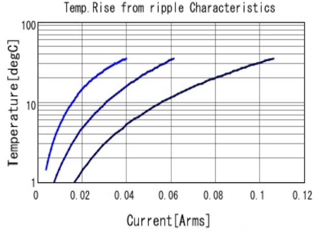
GRM21AR72E102KW01 Temp. rise ■ 30kHz ■ 100kHz ■ 300kHz
