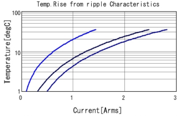
GRM21AR72A334KAC5 Temp. rise — 100kHz — 500
