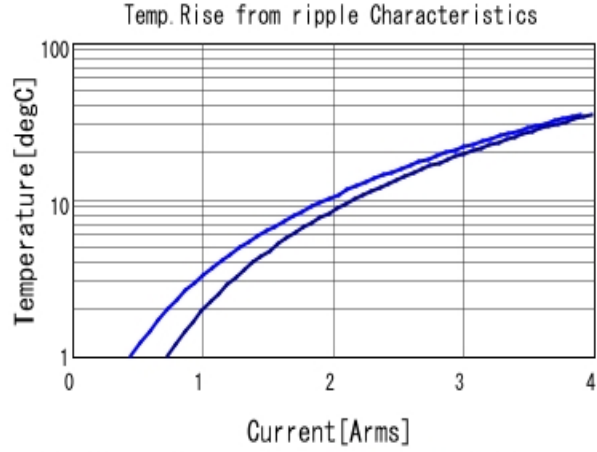
GRM219R61E225KA12 Temp. rise ■ 500kHz ■ 1MHz
