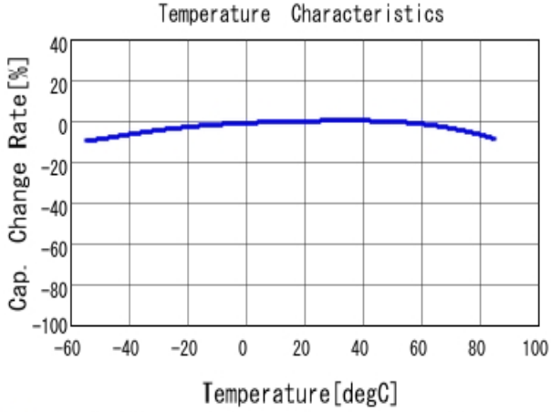
■ GRM219R61A106KE44 C-Temp. capchange, DCO. 0V, ACO. 5Vrm
