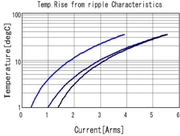
GRM219R61A106KE44 Temp. rise ■ 80kHz ■ 400kHz ■ 800kHz
