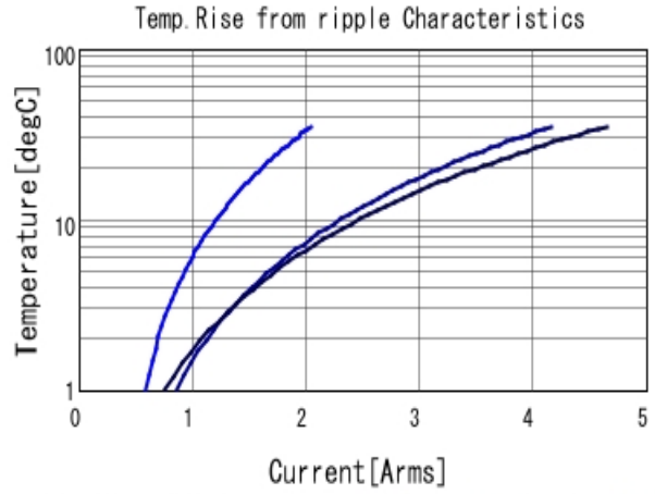
GRM219R61A105KA01 Temp. rise ■ 100kHz ■ 500kHz ■ 1MHz
