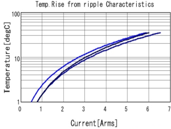
GRM219R60J226ME47 Temp. rise ■ 80kHz ■ 400kHz ■ 800kHz
