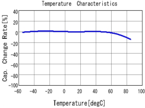
■ GRM219R60J226ME47 C-Temp. capchange, DCO. 0V, ACO. 5Vrm
