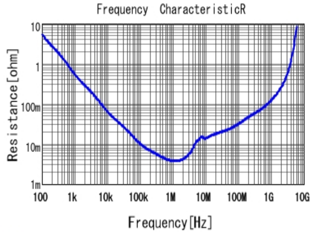
■ GRM219R60J106KE19 R DCOV, 25degC
