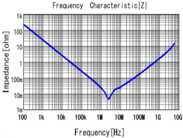
■ GRM219R60J106KE19 |Z| DCOV, 25degC
