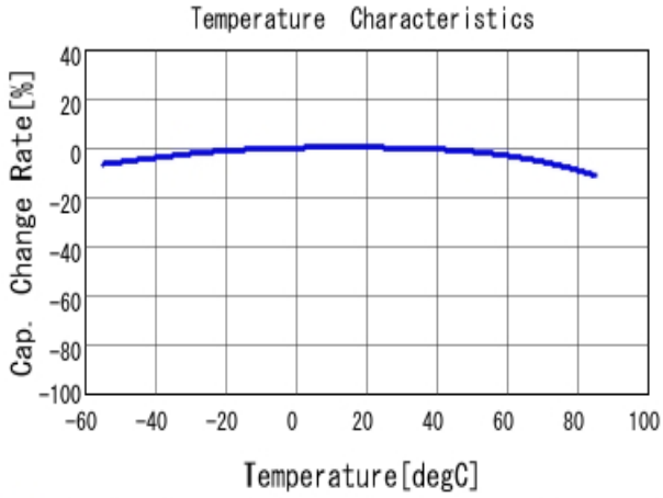
■ GRM219R60J106KE19 C-Temp. capchange, DCO. 0V, ACO. 5Vrm
