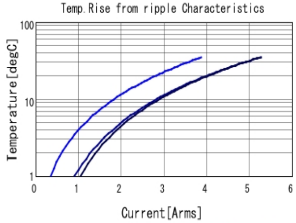
GRM219R60J106KE19 Temp. rise ■ 80kHz ■ 400kHz ■ 800kHz
