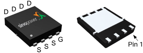
DFN5x6-8 (Punch-EP)
