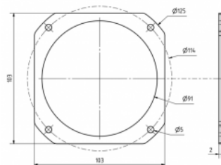
Dichtring/Gasket FRS 10 WP 22.04.2020
