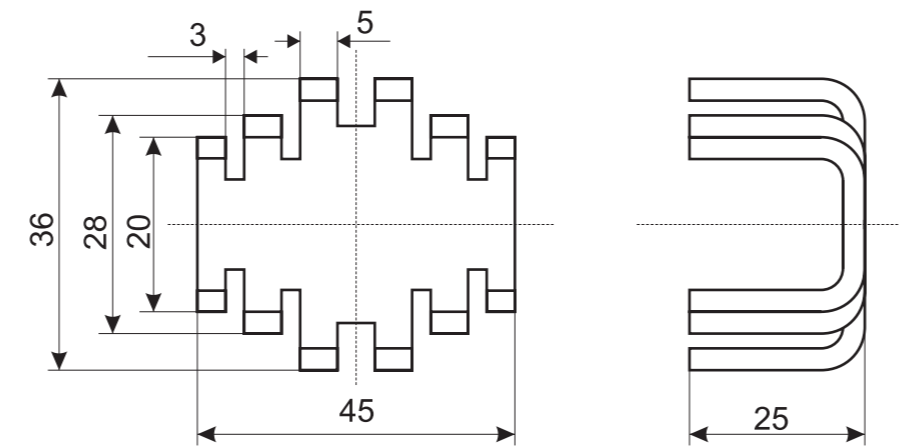
302 36x45x25 mm
