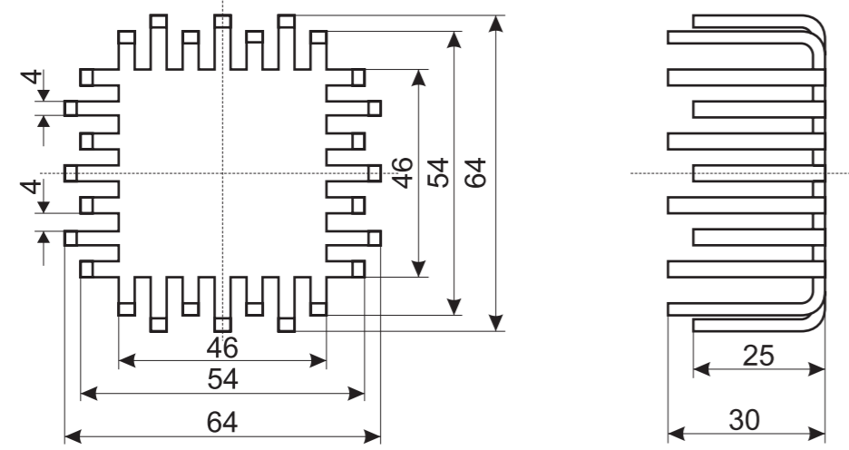
104 64x64x30 mm
