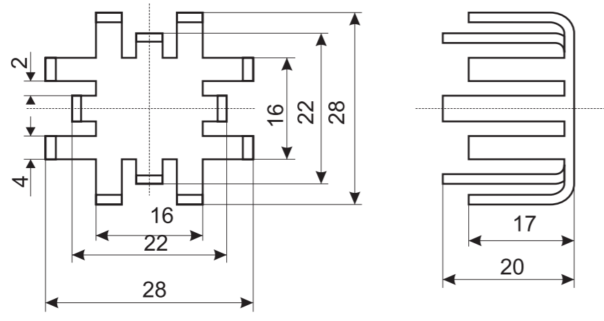
101 28x28x20 mm
