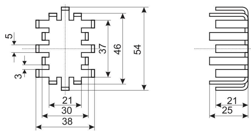
201 38x54x25 mm
