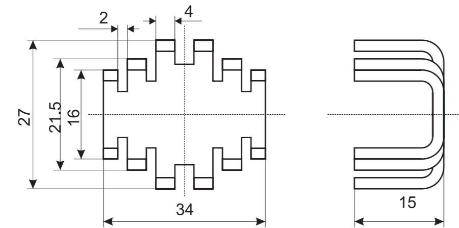
301 27x34x15 mm
