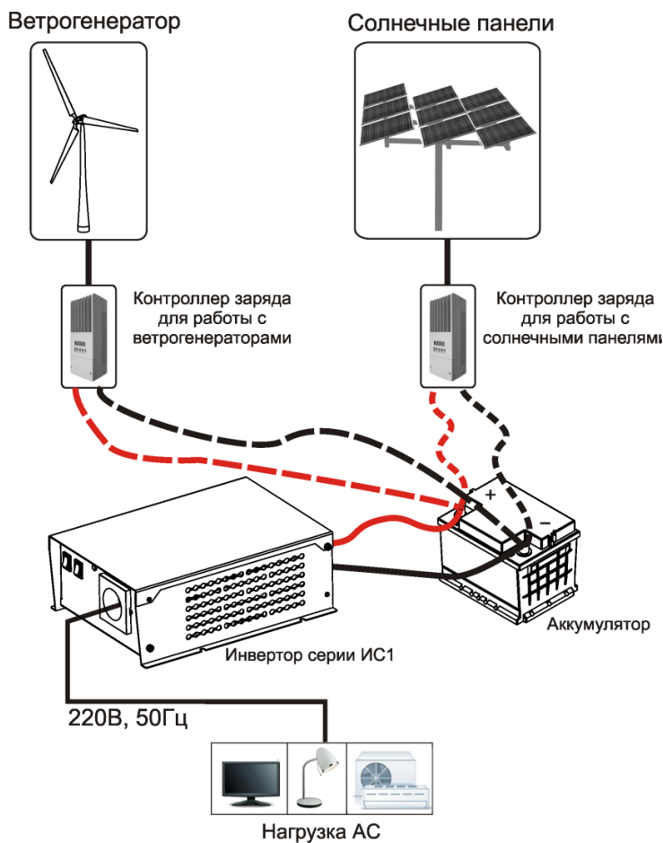
Рис.3 Схема подключения инверторов серии ИС1-У/У1/У2 к системам альтернативной энергетики
