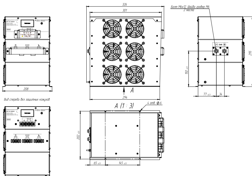
Рис.1.2 ИС1-24-6000У1 (вид изделия)
