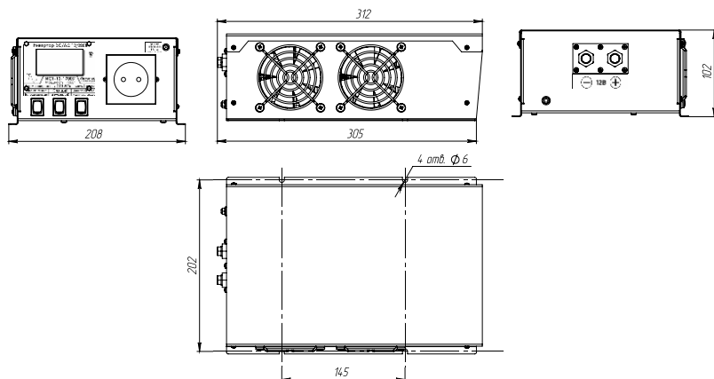
Рис.1 ИС1-12-1700У и ИС1-24-2000У (вид изделия)
