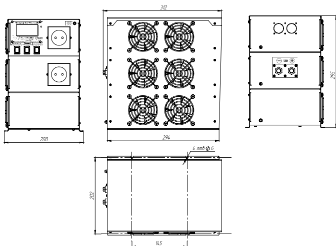
Рис.1.1 ИС1-24-6000У (вид изделия)
