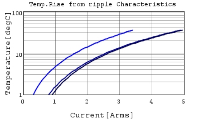
GRM319R61C106KE15 Temp.rise — 80kHz —
