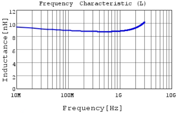
LQW15AN9N1H00 L
