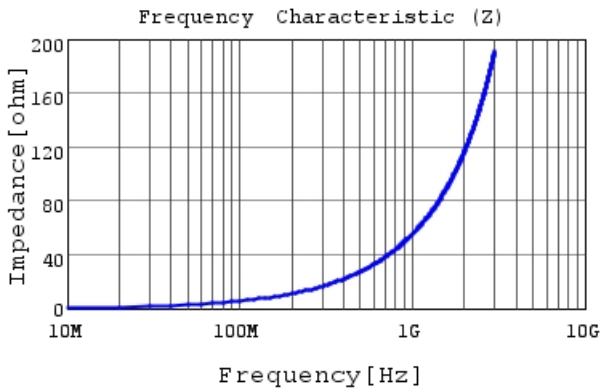
LQW15AN9N1H00 |Z|
