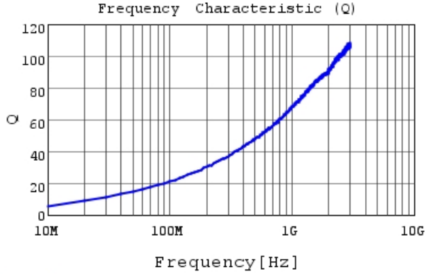
LQW15AN9N1H00 Q
