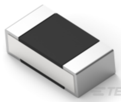
TE Part #9-2176307-8 RP 1E 0.1W 127K 0.1% 25PPM 5K RL
