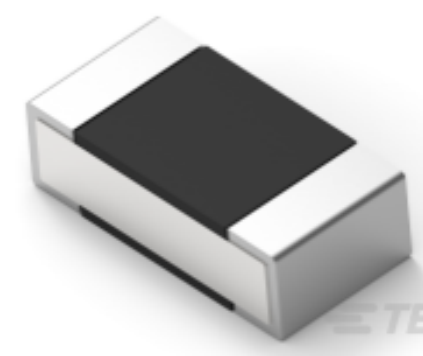
TE Part #2176308-3 RP 1E 0.1W 140K 0.1% 25PPM 5K RL
