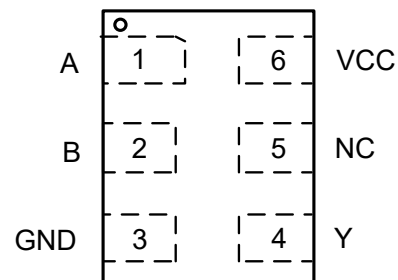
DFN6(1×1.5)
