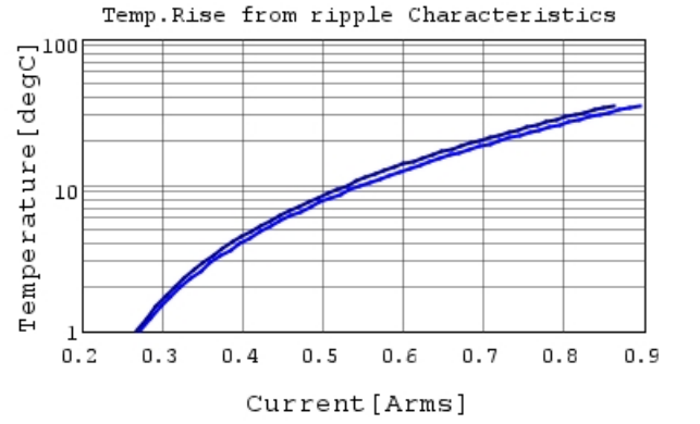
GJM1555C1H2R0CB01 Temp.rise — 2GHz — 3
