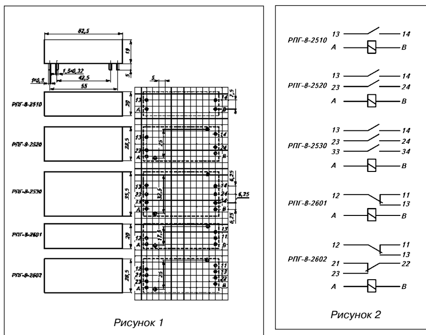
Рис. 1. Габаритные и установочные размеры реле РПГ-8
