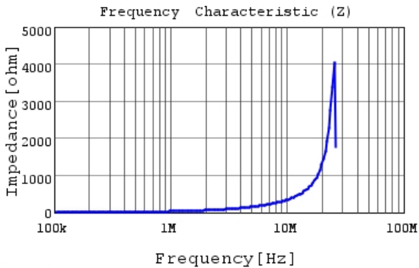
1277AS-H-4R7M |Z|
