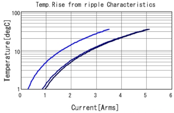
GRT188R61A106KE13 Temp. rise ■ 80kHz ■ 400kHz ■ 800kHz
