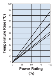
RK73H 2A-2E
