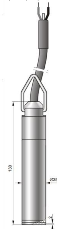
Dimension - Dimensión
