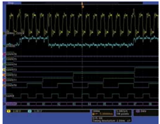
Рис. 16. MSO имеет 16 встроенных цифровых каналов, позволяя отображать и анализировать коррелированные по времени аналоговые и цифровые сигналы.
