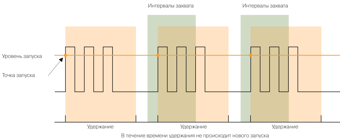
Рис. 35. Удержание запуска
