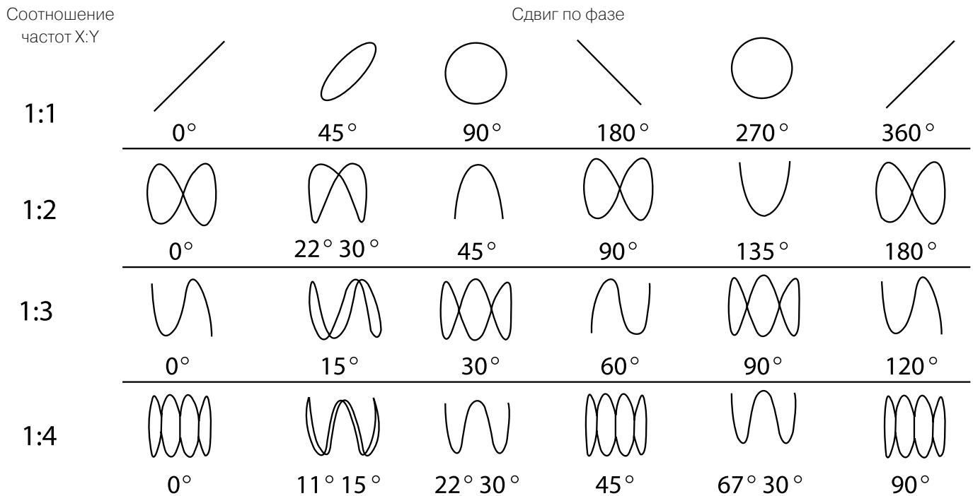
Рис. 69. Фигуры Лиссажу
