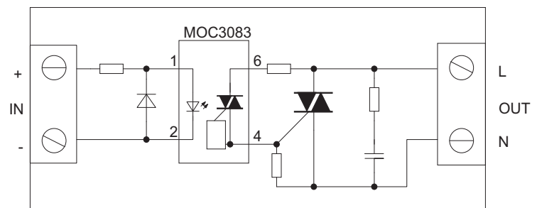
Рис. 2. Схема модуля
