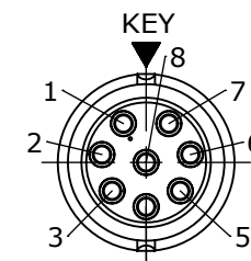
WIRING END W6280-8SG-P-5XX
