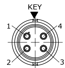
WIRING END W6280-4SG-P-5XX
