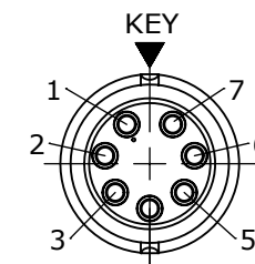
WIRING END W6280-7SG-P-5XX
