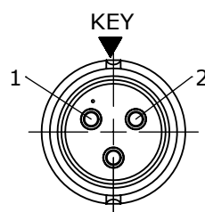
WIRING END W6280-3SG-P-5XX
